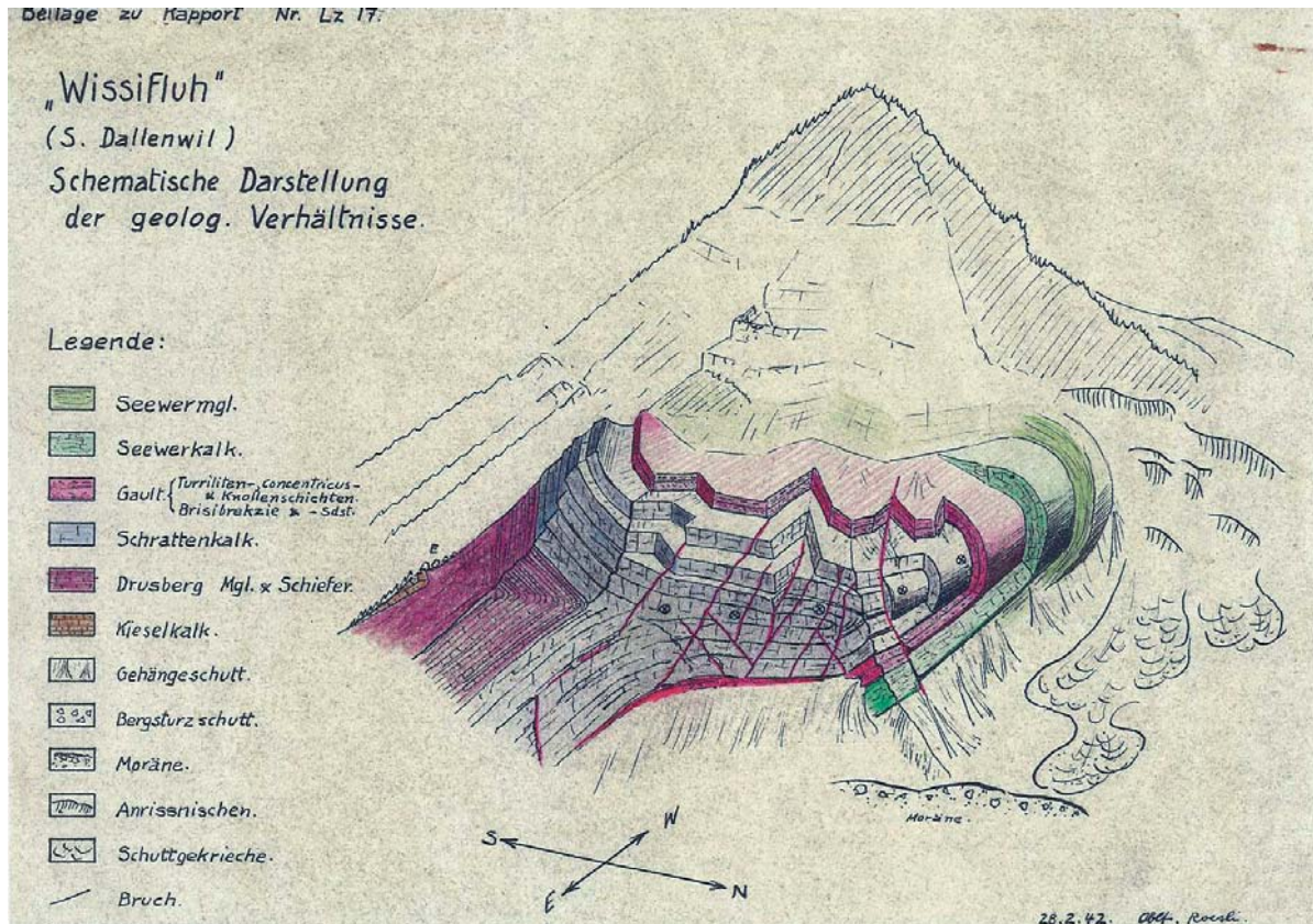
Fig. 2: Geologische Aufriss-Zeichnung der Wissifluh, NW. Von Franz Roesli (1942 b). Diese Abbildung ist bereits in der Offiziersgesellschaft Nidwalden (2007, Fig. 89, S. 79) reproduziert worden.
