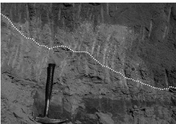
Fig. 5: Einschnitt Tunnelbaustelle Neufeld. Detail von Fig. 4. Grobkörniges Sediment (Konglomerate mit mud pebbles, sog. lag) über erosiver Basis einer Rinne (gestrichelte Linie). Foto: Bernhard Hostettler (NMBE).
