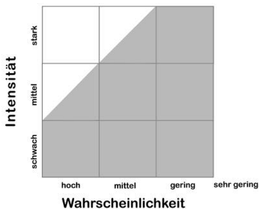
Fig. 3: Waldwirkung gegenüber Stein- und Blockschlag, dargestellt im Intensitäts-Wahrscheinlichkeits-Diagramm des Bundes (BRP, BWB, BUWAL 1997). Gute bis sehr gute Wirkungen im Bereich schwacher und mittlerer Intensität; im Bereich starker Intensität nur mehr bei seltenen Ereignissen. Bei häufigen Ereignissen starker Intensität wird der Wald zerstört und kann gar nicht mehr oder nur in Form einer wenig wirksamen Pionierphase überdauern.
