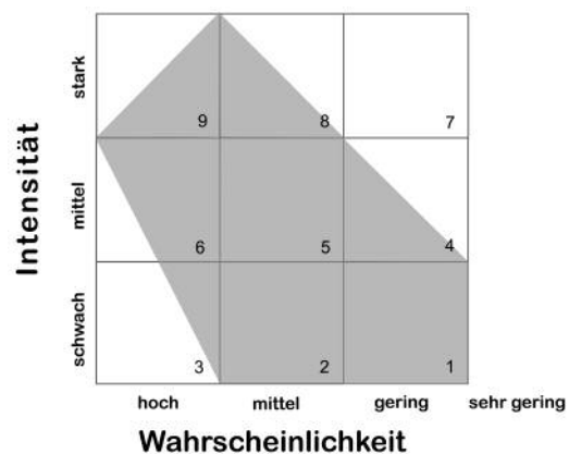
Fig. 4: Waldwirkung gegenüber Rutschungen, Erosion und Hangmuren, dargestellt im Intensitäts-Wahrscheinlichkeits-Diagramm des Bundes (BRP, BWB, BUWAL 1997). Gute bis sehr gute Wirkungen im Bereich schwacher und mittlerer Intensität. Wenig Wirkung im Bereich der tiefgründigen, permanenten Rutschungen (Feld 3) und der mittel- bis flachgründigen, spontanen Hangmuren (Felder 7, 8). Eingeschränkte Wirkung im Bereich ständiger, starker Bodenbewegungen (Feld 9), wo sich vielfach keine oder nur noch eine Pionierbestockung halten kann.
