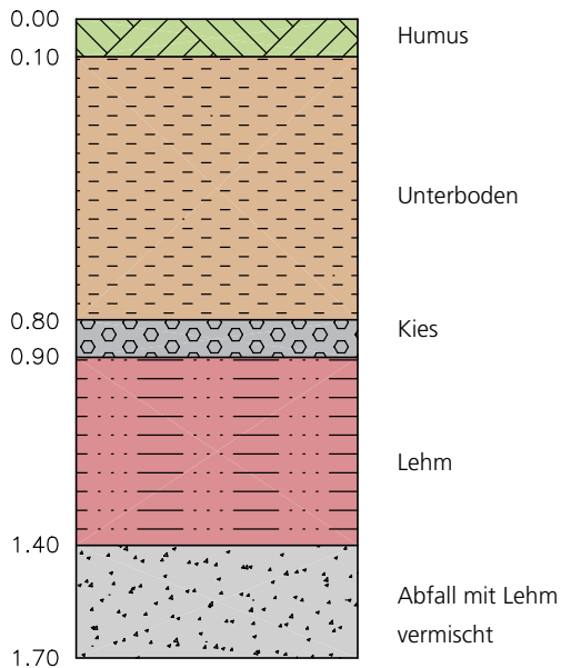
Fig. 2: Typischer Aufbau des Deponiekörpers. Rechts: Blick in einen Sondierschacht; links: Schematisches Profil aus dem selben Schacht.
